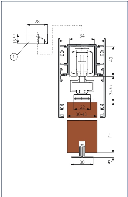
Wand- / Takmontering tre med klipsdeksel 100, på begge sider
