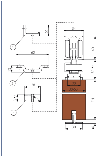
Wand- / Takmontering tre
