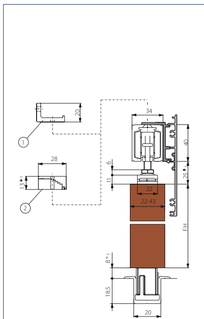
Vegg- / takmontering tre med avstandsholder og klipsdeksel 100
