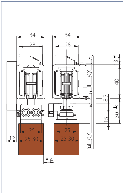
Takmontering tre med klipsdeksel 100
