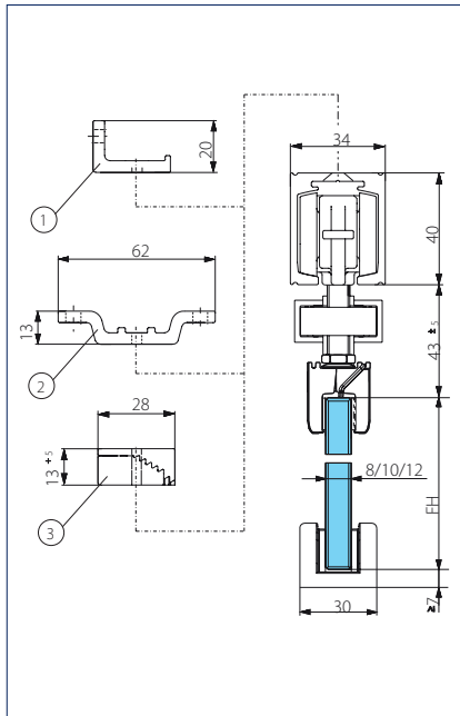
Vegg- / takmontering glass med glass-klemmeplate 30
