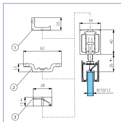
Perlan med glassklemmeplate 30 mm
