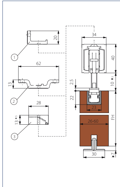
Vegg- / takmontering skjult opphengsprofil
