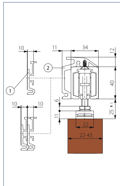
Veggmontering tre med skjult veggfeste
