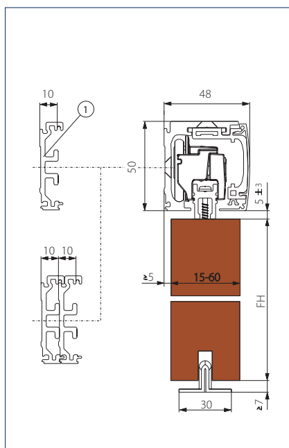
Veggmontering tre
