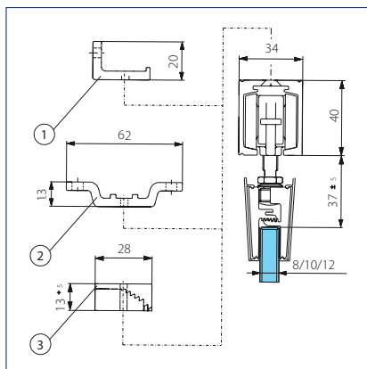
Perlan med glassklemmeplate 45
