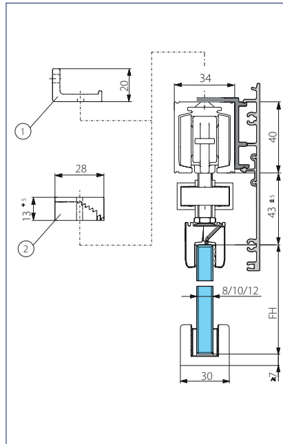
Vegg- / takmontering glass med glass-klemmeplate 30 og klipsdeksel 100, ensidig
