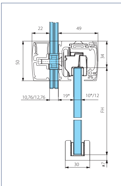
Overlysmøntering glass
