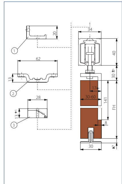
Wand- / Takmontering tre
