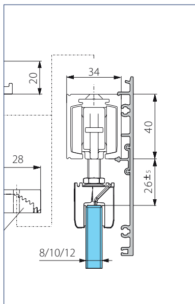
Vegg- / takmontering glass med glass- klemmeplate 30 og klipsdeksel 100 FH = Fløyhøyde 1 = Veggfeste 2 = Høydeutjevning
