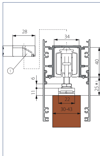
Vegg- / takmontering tre med avstands- holder og klipsdeksel 100 1 = Veggfeste 2 = Høydeutjevning
