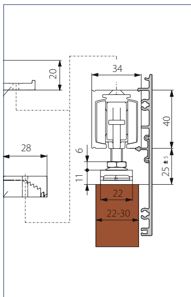
Wand- / Takmontering tre med klipsdek- sel 100 1 = Veggfeste 2 = Høydeutjevning
