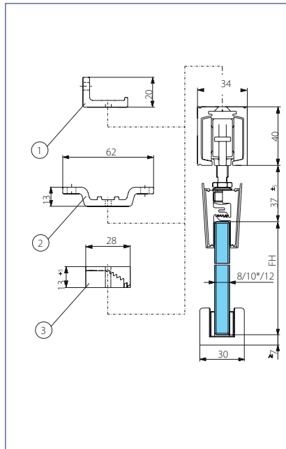
Vegg- / takmontering glass med glass- klemmeplate 45 og gjennomgående deksel
