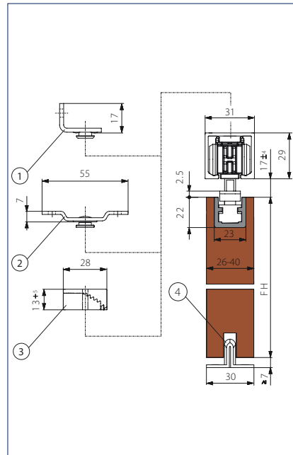
Vegg- / takfeste tre med skjult bæreplate
