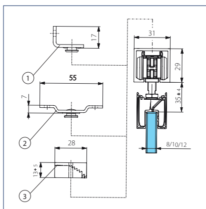
Rollan med glassklemmeplate 30 mm
