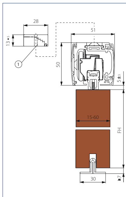
Takmontering tre
