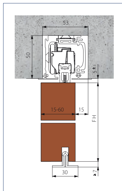
Takmontering skjult tre
