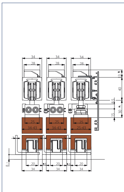
Takmontering tre med avstandsholder og klipsdeksel 100
