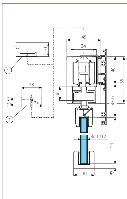
Vegg- / takmontering glass med klipsdeksel 100, ensidig
