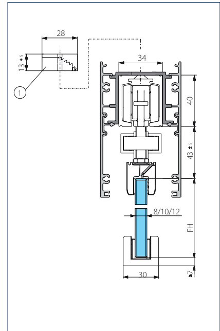
Vegg- / takmontering glass med glass-klemmeplate 30 og klipsdeksel 100, på begge sider
