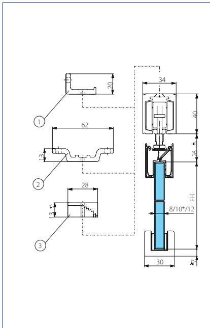
Vegg- / takmontering glass med glass- klemmeplate 30 og gjennomgående deksel
