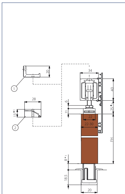
Wand- / Takmontering tre med klipsdeksel 100, ensidig
