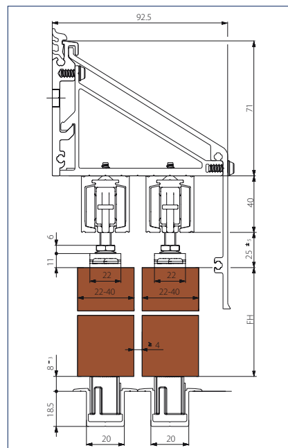
Vegg- / takmontering tre med Perlan veggfeste og værdeksel
