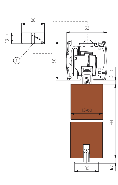
Takmontering tre
