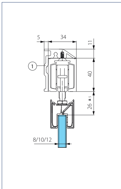
Veggmontering glass med skjult veggfeste og glassklemmeplate 30, gjennomgående dekket
