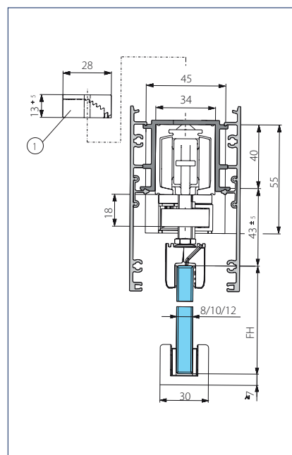
Vegg- / takmontering glass med klipsdeksel 100, på begge sider
