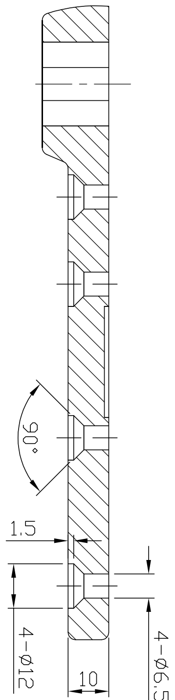
Door Shoe
