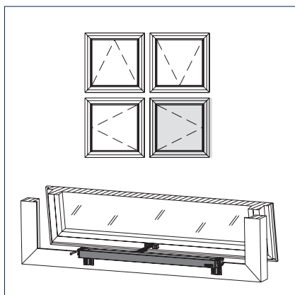
ÅPNING UTOVER rammemontering
