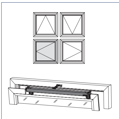
ÅPNING INNOVER vindusrammemontering
