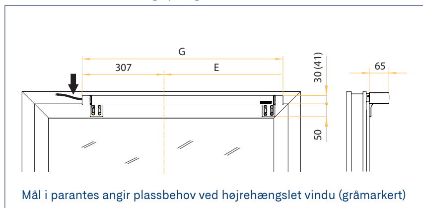
Plasskrav for vindusrammemontering åpning INNOVER
