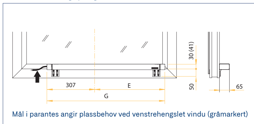
Plasskrav for rammemontering åpning UTOVER
