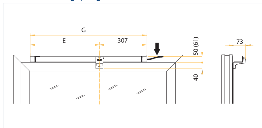
Plasskrav for rammemontering åpning INNOVER
