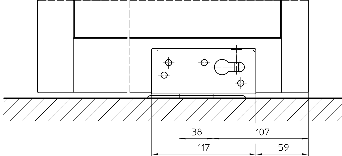
Vorderansicht: Bodenschloß, rechts schließend Front view: Floor lock, right closing
