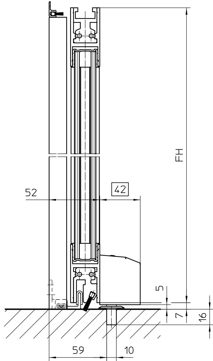
V: Bodenschloß, Winkelbodenführung V: Floor lock, angular floor guide
