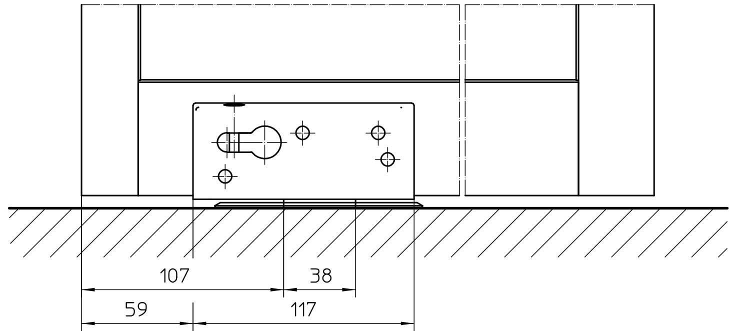
Vorderansicht: Bodenschloß, links schließend Front view: Floor lock, left closing
