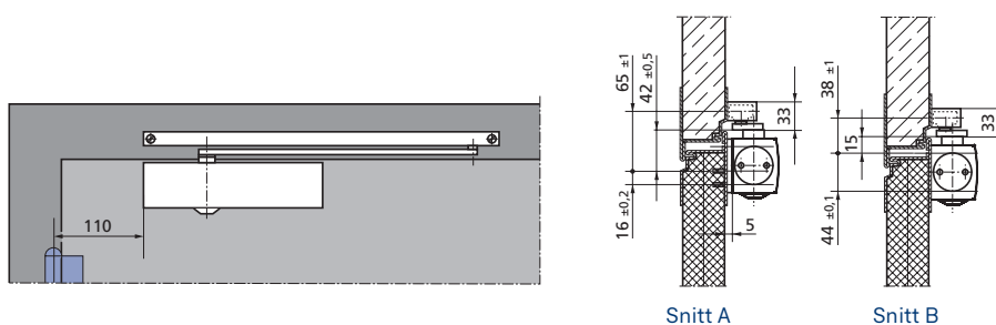
Snitt A
