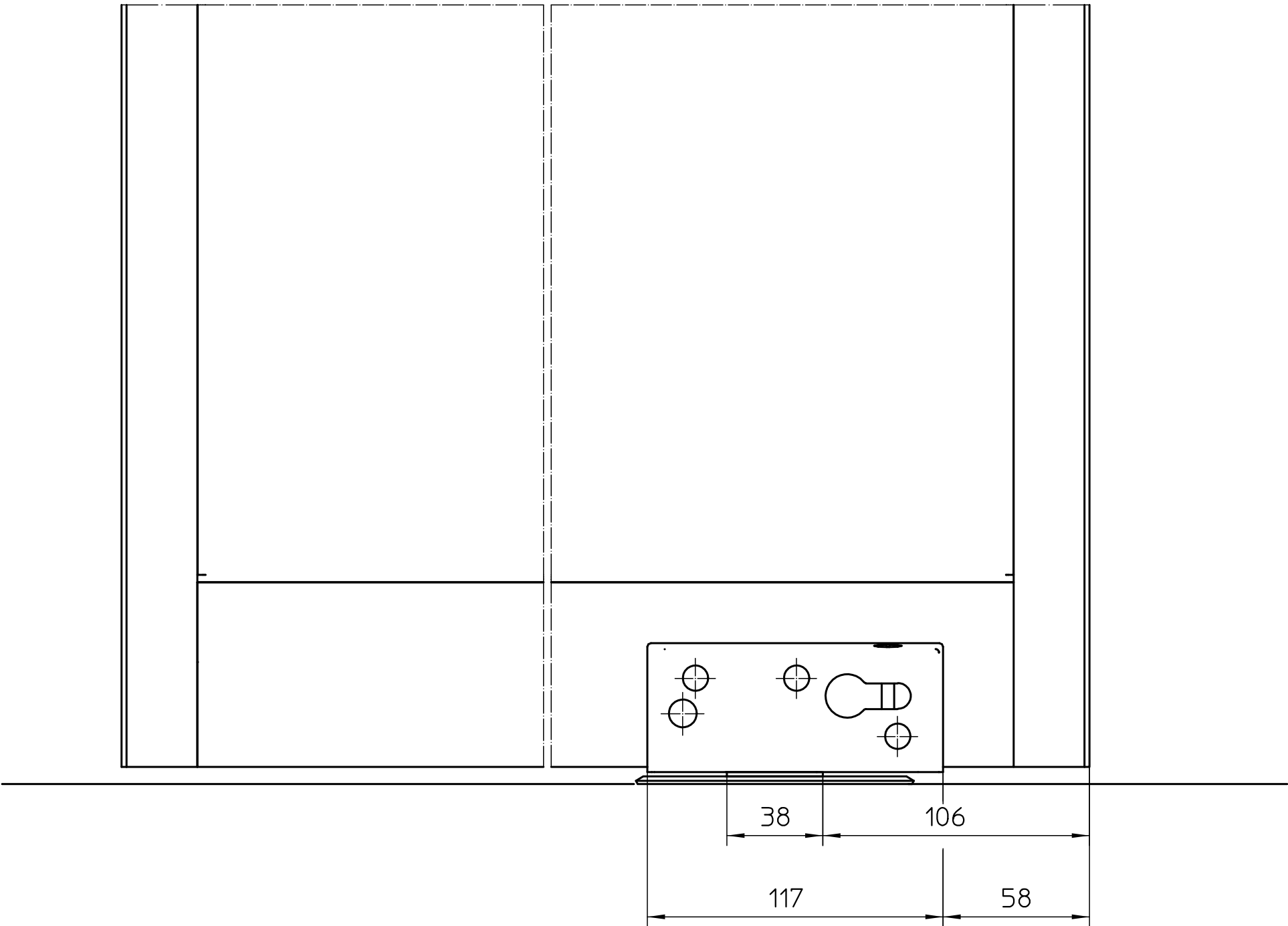
Vorderansicht: Bodenschloß, recht schließend Front view: Floor lock, right closing
