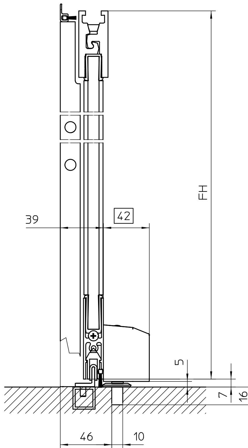
V: Bodenschloß, Winkelbodenführung V: Floor lock, angular flor guide
