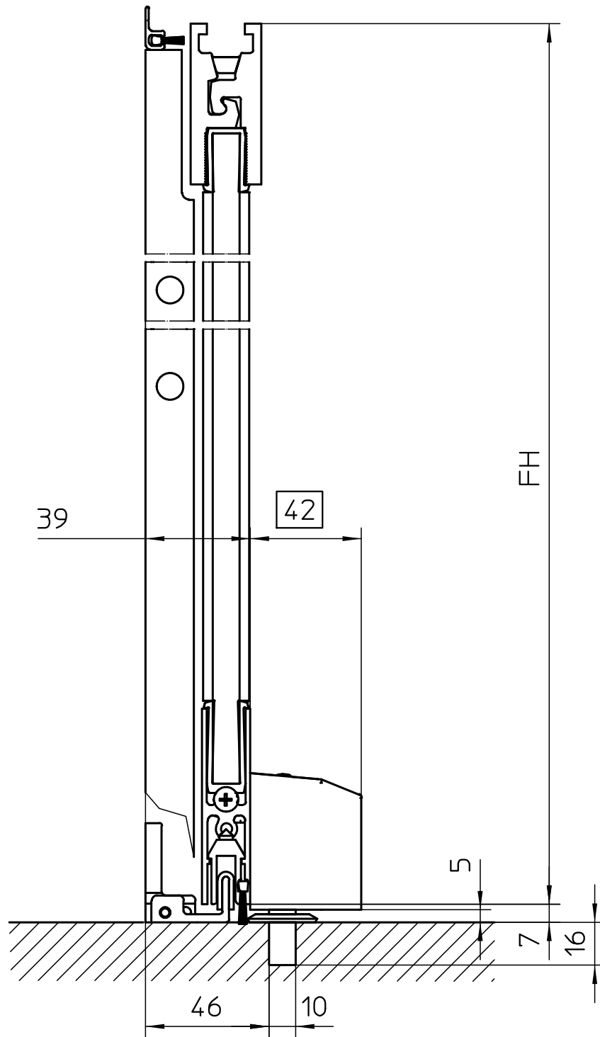
V: Bodenschloß, Winkelbodenführung V: Floor lock, angular flor guide
