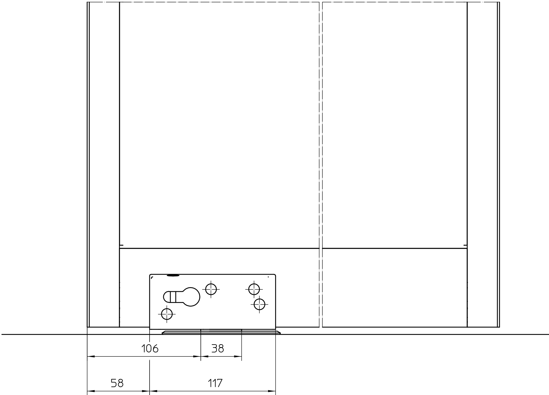
Vorderansicht: Bodenschloß, links schließend Front view: Floor lock, left closing
