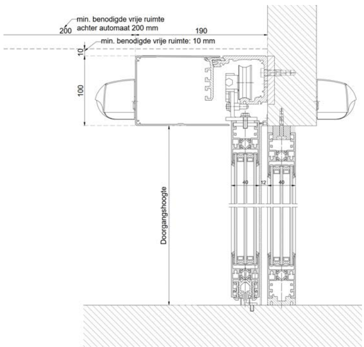
Verticale doorsnede
