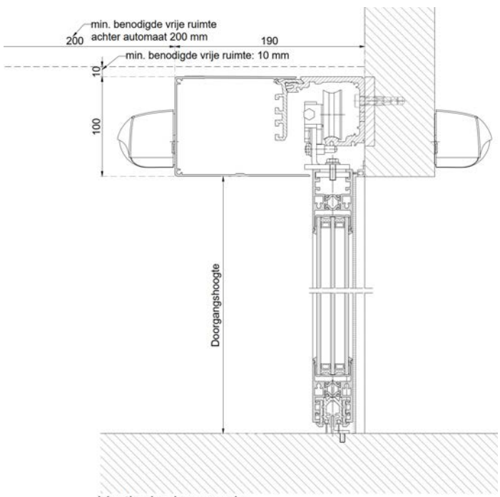
Verticale doorsnede
