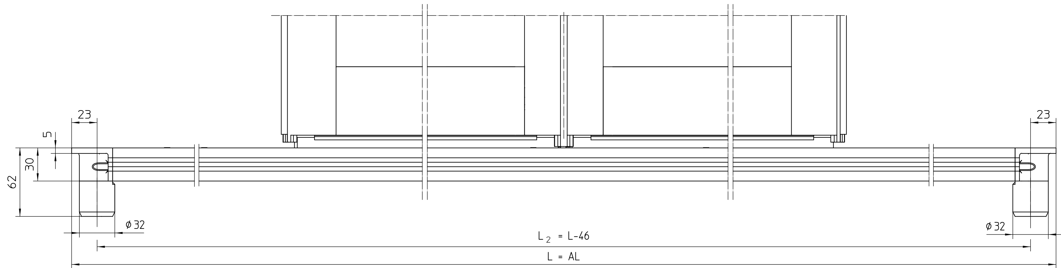
H: Horizontalschnitt mit Wand H: horizontal section with wall
