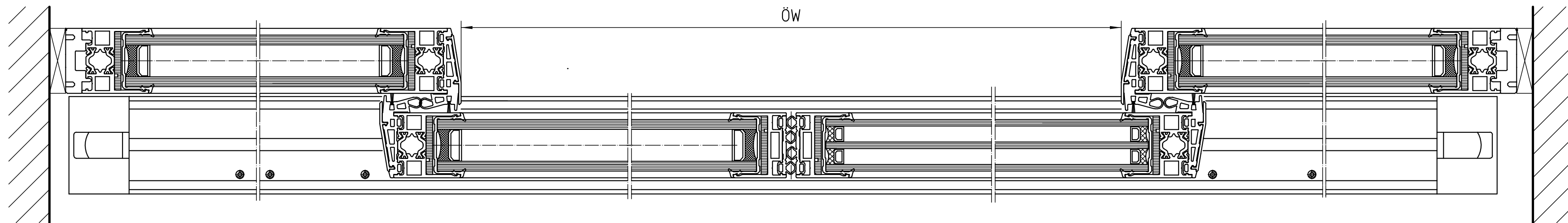
H: Horizontalschnitt mit Seitenteil unter Träger H: horizontal section with fixed leaf below girder
