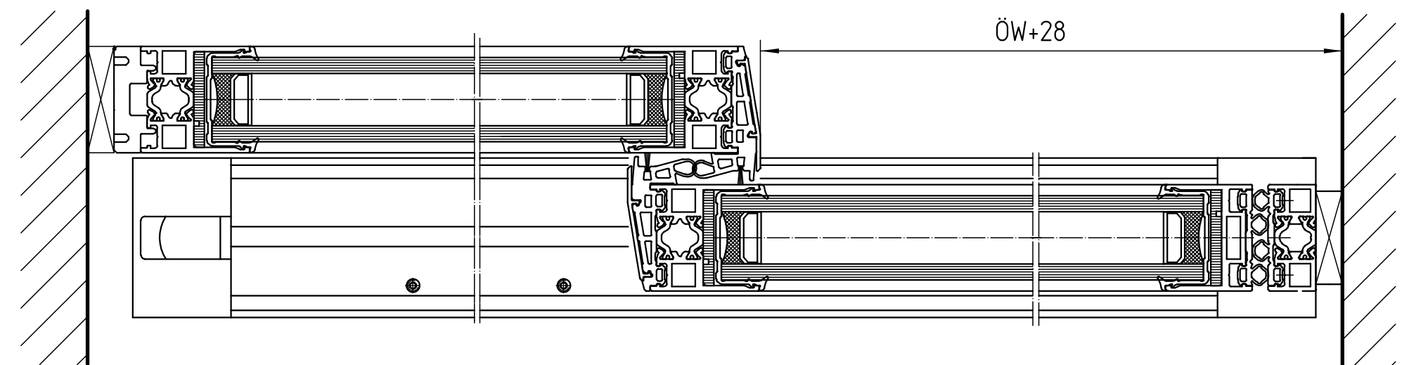
H: Horizontalschnitt mit Seitenteil unter Träger H: horizontal section with fixed leaf below girder
