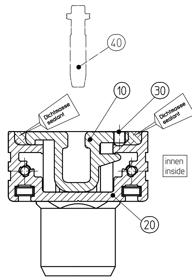
V: Vertikalschnitt mit Seitenteil V: vertical section with side panel
