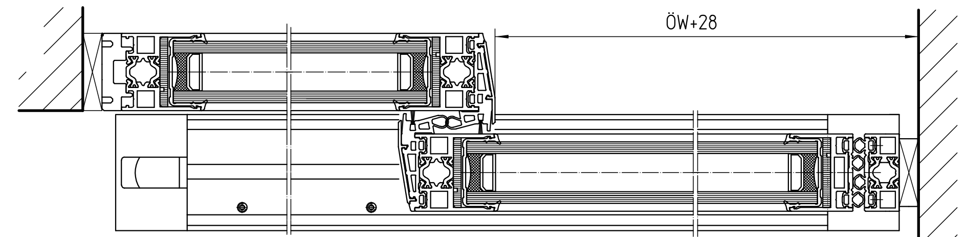
H: Horizontalschnitt mit Seitenteil unter Sturz H: horizontal section with fixed leaf below lintel
