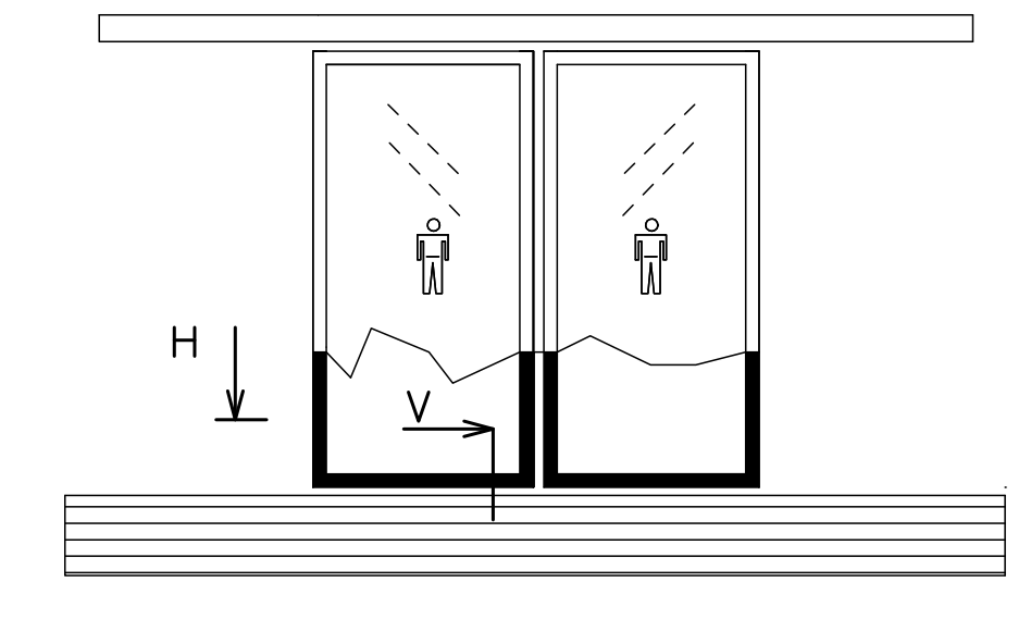
H-V: Unterer Türabschluß H-V: Bottom attachment
