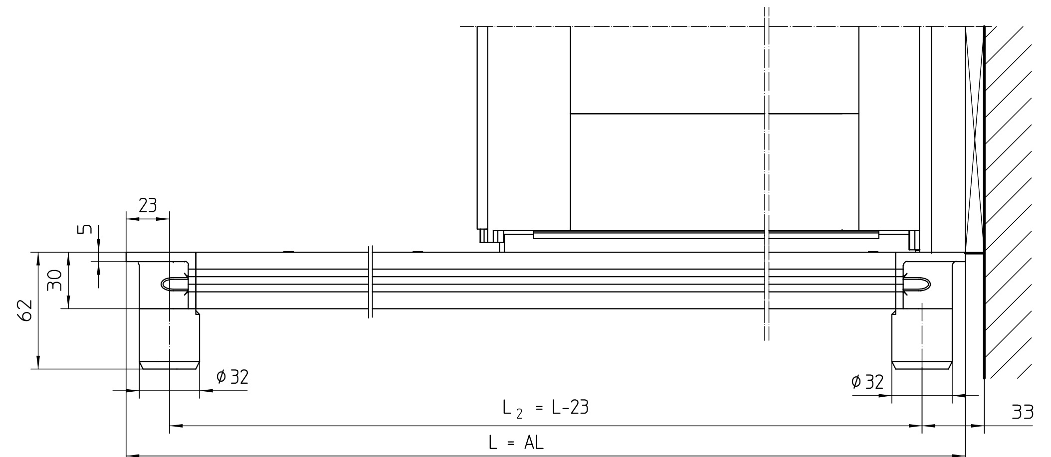
H: Horizontalschnitt mit Wand H: horizontal section with wall
