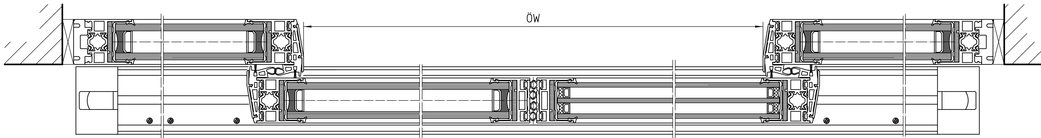
H: Horizontalschnitt mit Seitenteil unter Sturz H: horizontal section with fixed leaf below lintel
