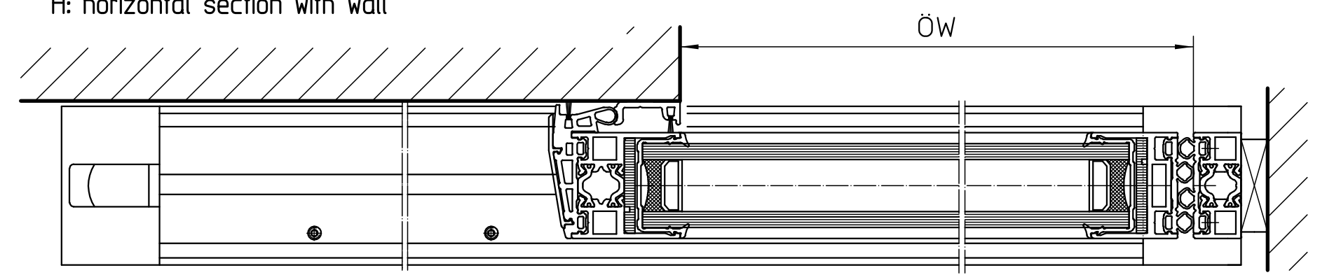
H: Horizontalschnitt mit Wand H: horizontal section with wall
